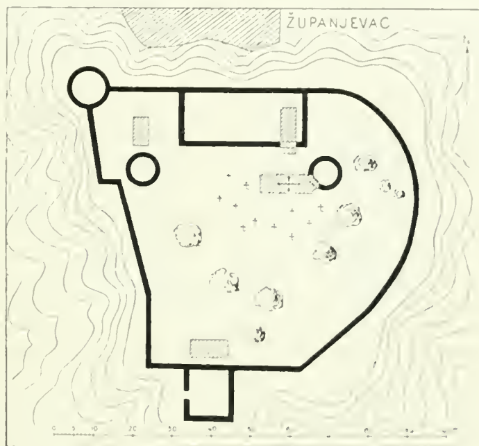
ŽUPANJEVAC, Kastellplan.
