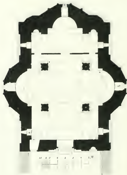
RAVANICA, Grundriss der Kirche
