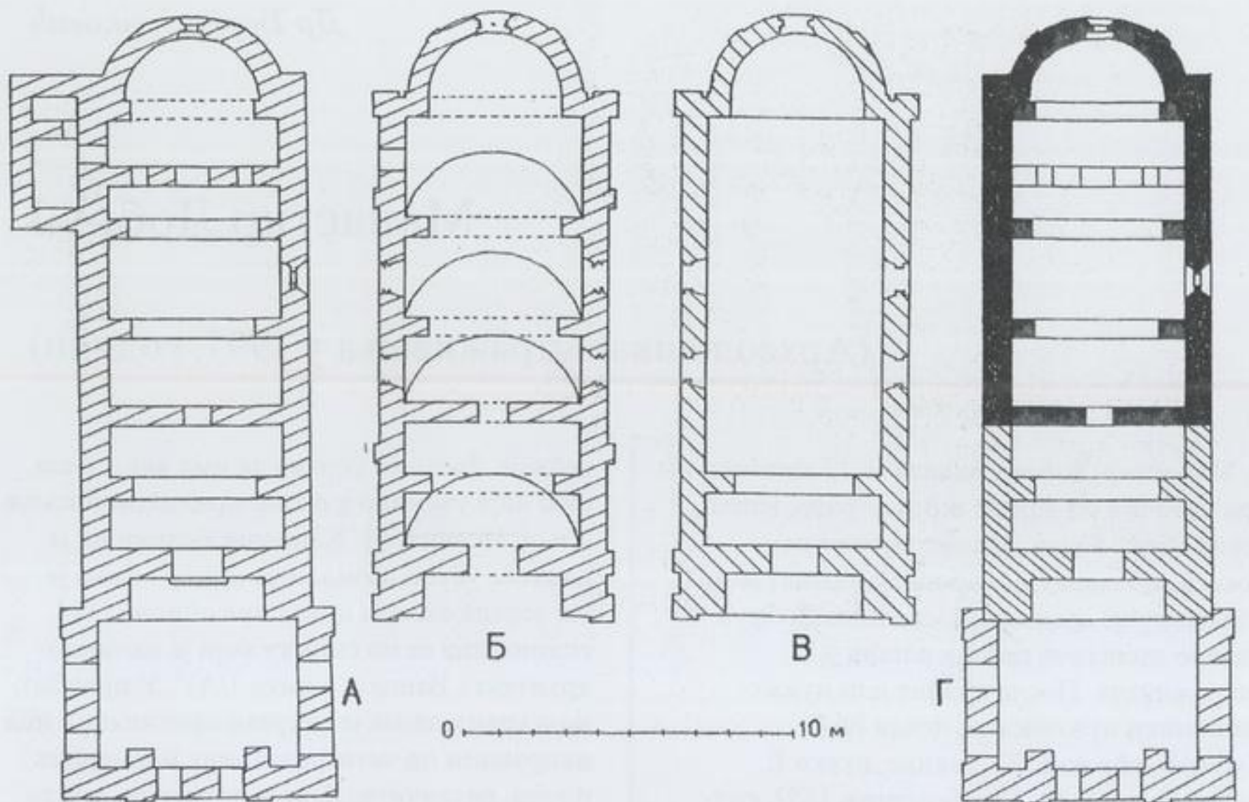
Слика 1. Основа храма посвећеног Благовештењу из 1884. (А) и 1928. (Б) по М. Кашанину; приближна основа храма данас (В) и претпостављене фазе грађења (Г)
