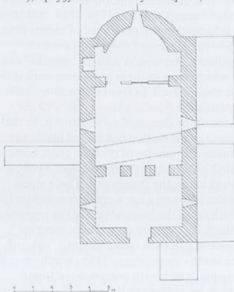
Сл. 3 Основа цркве Св. Димитрија са уцртаним сондама
